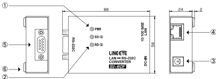
SI-60F 標準モデル (型番: SI-60F)
