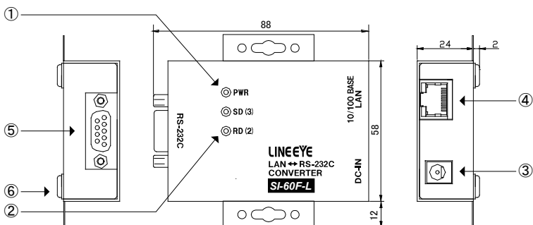
SI-60F 壁掛モデル (型番: SI-60F-L)
