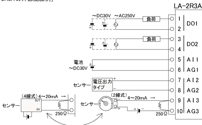
[LA-2R3A の外部配線例]
