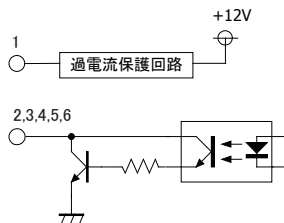
オープンコレクタ出力回路
