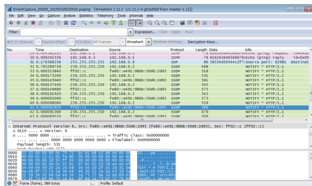
[ Wiresharkによる解析表示画面 ]
