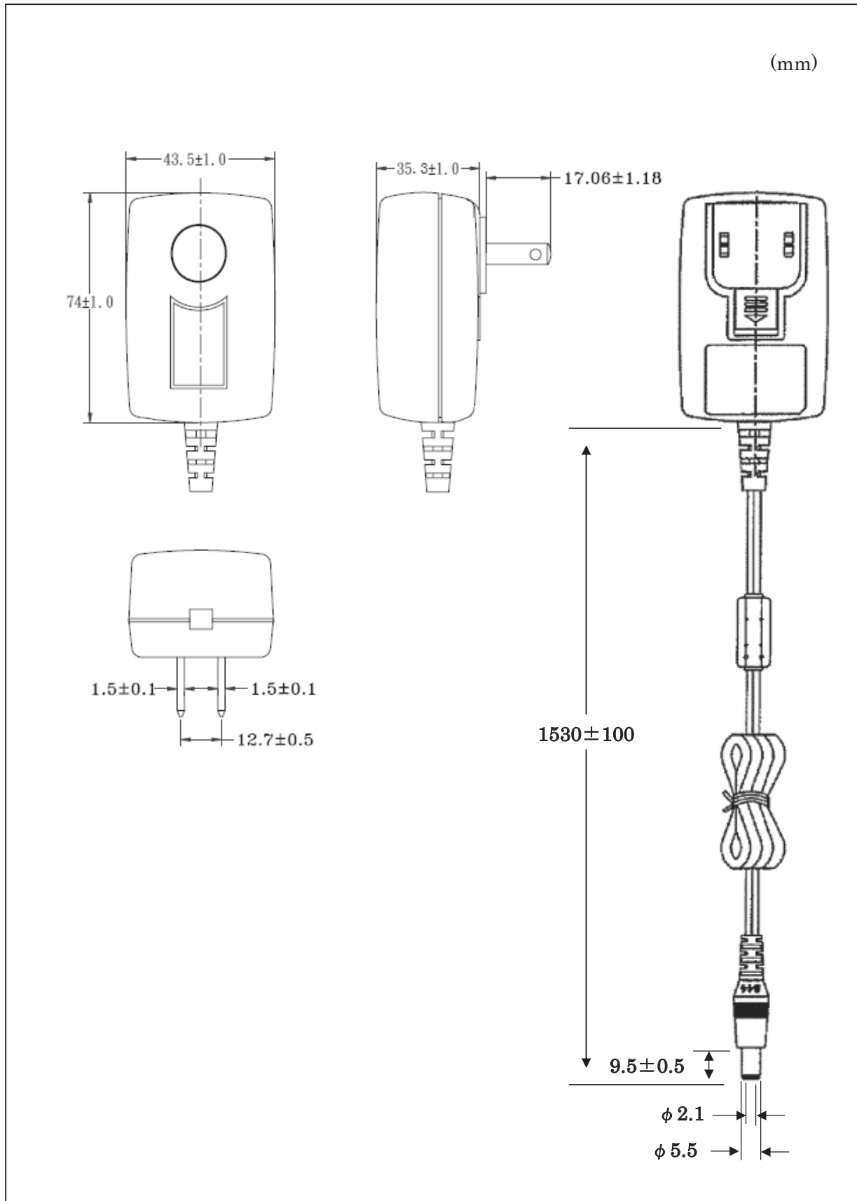
ワイド入力ACアダプタ外形図 型番：6A-181WP09
